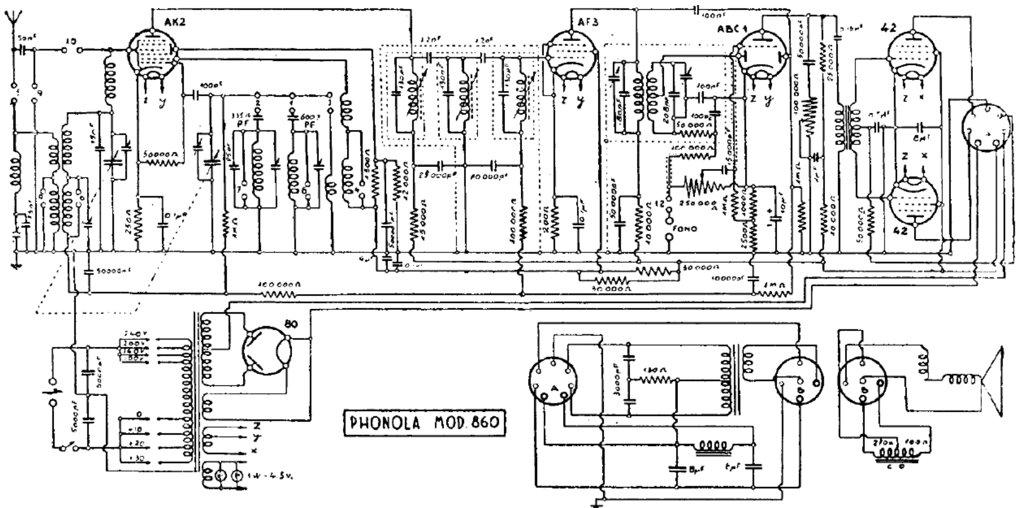
PHONOLA (S. A. FIMI). — Modelli « 860, 861 e 863 ». - Produzione 1937. - Media frequenza: 470 kHz.
